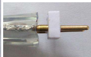
Widok z przekroju po mocowaniu 2-piniowego łącznika
