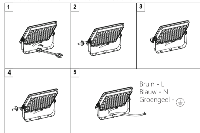
DEMONTAGESHEMA LICHTBRON
